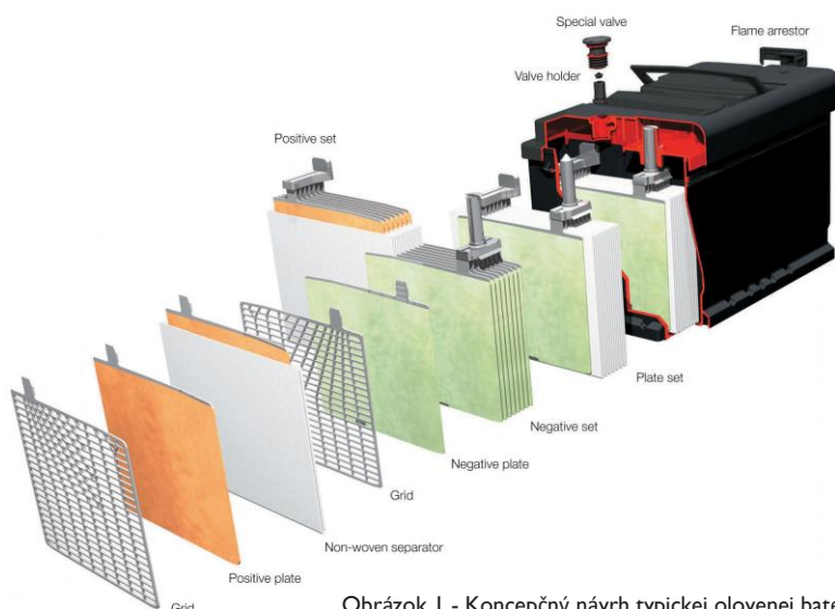
Obrázok I - Koncepčný návrh typickej olovenej batérie.
